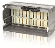
E6.2 W FP lu=5000 3p HR HR 1SDA073917R1
