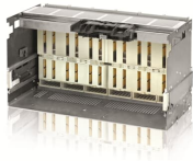
E6.2 W FP Iu=5000 3p HR HR 1SDA073917R1
