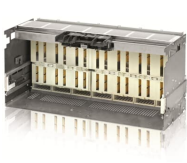
E6.2-A W FP 5000 4p HR HR 1SDA079707R1
